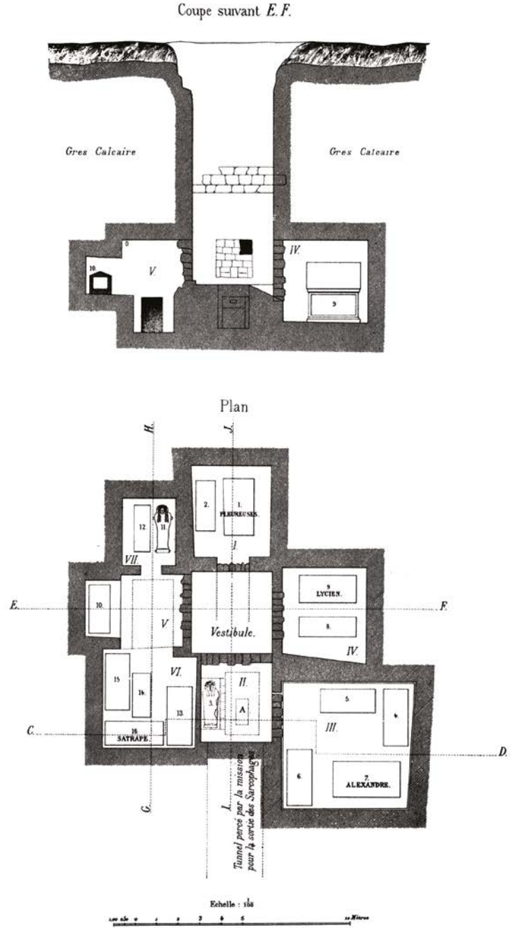
Fenike (Sidon) krallarına ait olduğu düşünülen hipojelerin plan ve kesitleri (üstte). Odalar ve içlerinde bulunan önemli eserler: 1. oda - Ağlayan Kadınlar Lahdi, 2. oda - Tabnit Lahdi, 3. oda - İskender Lahdi, 4. oda - Likya Lahdi, 6. oda - Satrap Lahdi, 7. oda - Antropoid lahitler.
